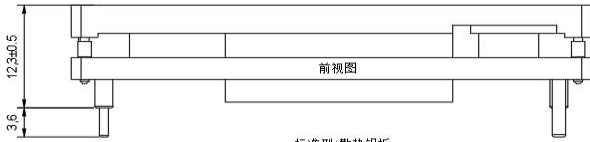
标准型+散热铝板 58.1mm*23.0mm*12.3mm
