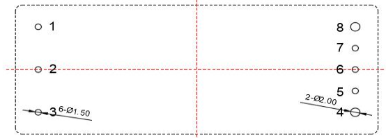
推荐PCB开槽尺寸
